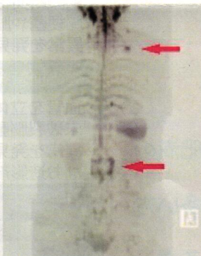
DWIBS画像
